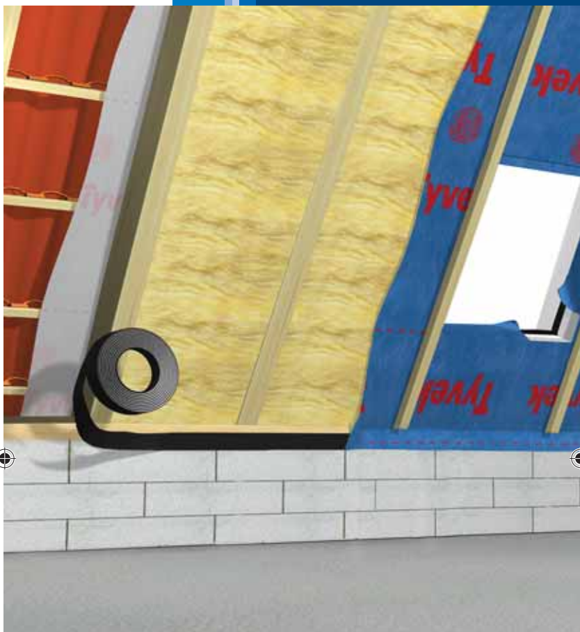
Рис. 10 Монтаж пароизоляции
