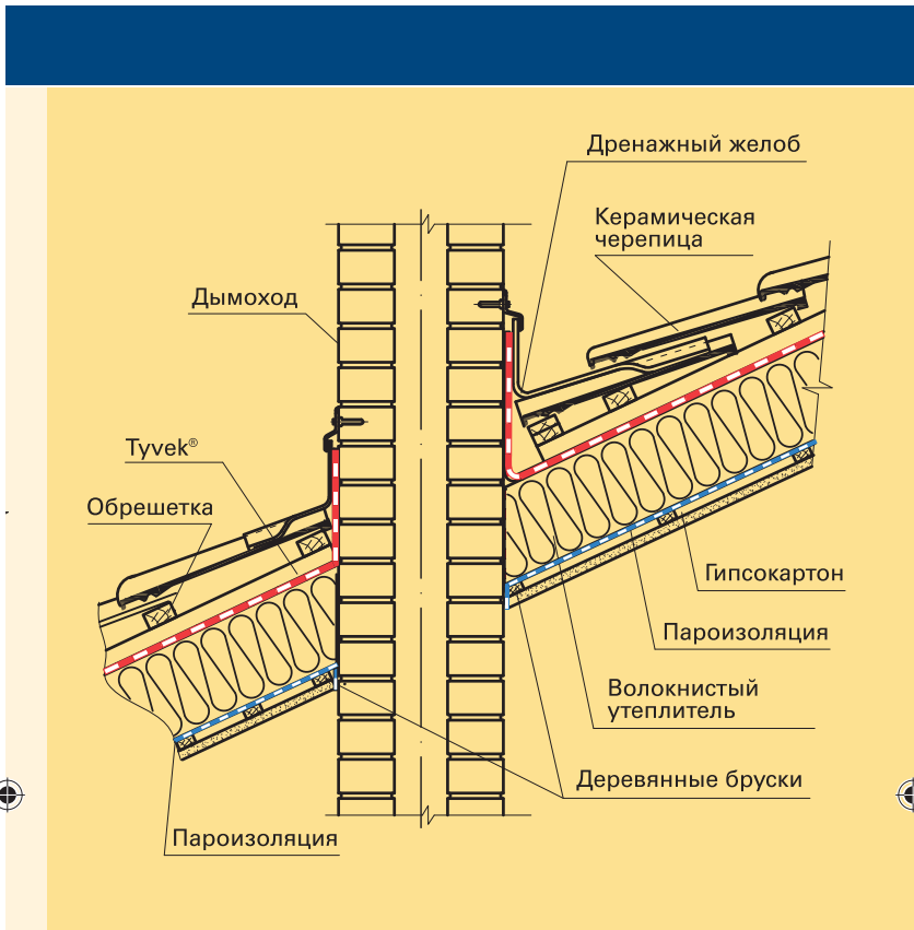
Рис. 3 Дымоход
