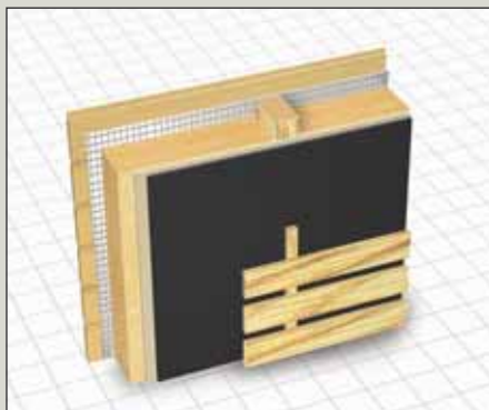
DELTA®-FASSADE/DELTA®-FASSADE PLUS
