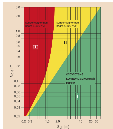
Зона диффузионных гидроизоляционных плёнок с высокой паропроницаемостью.
