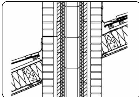
Проём для люка-лаза, печной или вентиляционной труб.
